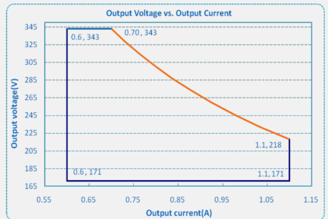
F1-240X-343
