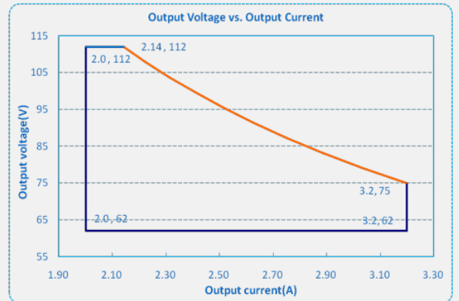
F1-240X-112
