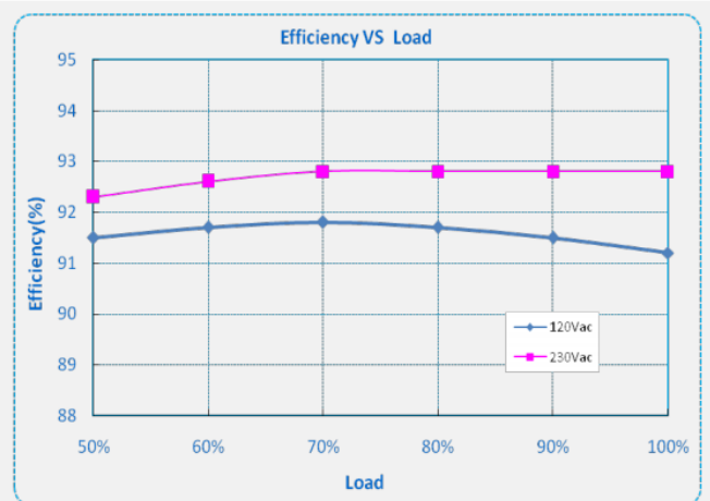
F1-240X112 ( I_o=2.22A )
