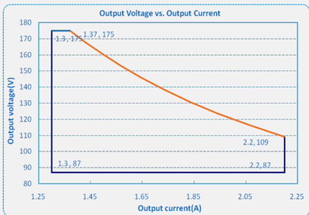
F1-240X-175
